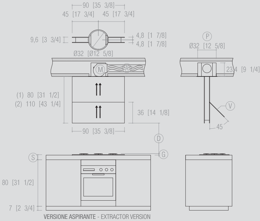
CAPPA SAIL (P) Diametro foro soffitto per incasso blocco motore (versione aspirante). (M) Portata di aspirazione motore cappa, pari a 1000 mc/h. (A) Tubo corrugato in alluminio ø 12 cm per fuoriuscita aspirazione fumi (versione aspirante). (D) Distanza minima griglie piano cottura - fondale cappa 55 cm. (G) Altezza griglie piano cottura. (S) Spessore piano di lavoro. (V) Sportello apribile per convoglio fumi al gruppo di aspirazione. (B) Feritoie per fuoriuscita aria filtrata (versione filtrante).
