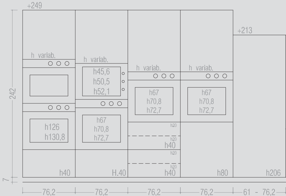
MODULARITA' BASI E COLONNE per elettrodomestici con standard americano: vista frontale.
