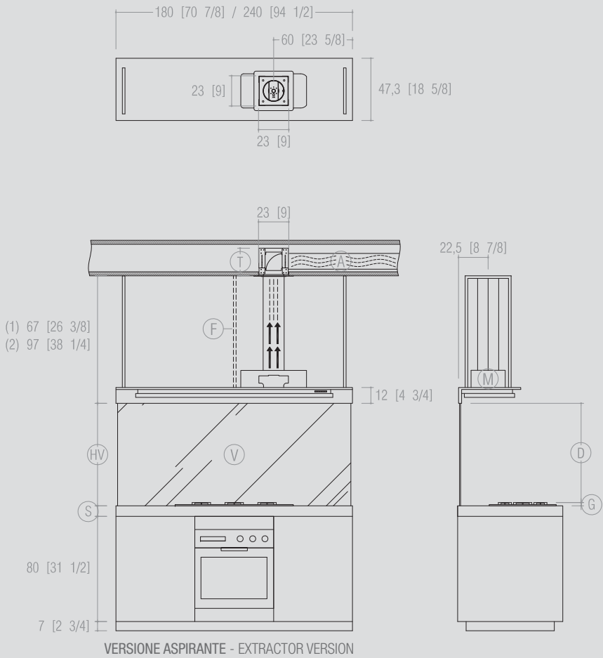
VERSIONE ASPIRANTE - EXTRACTOR VERSION
