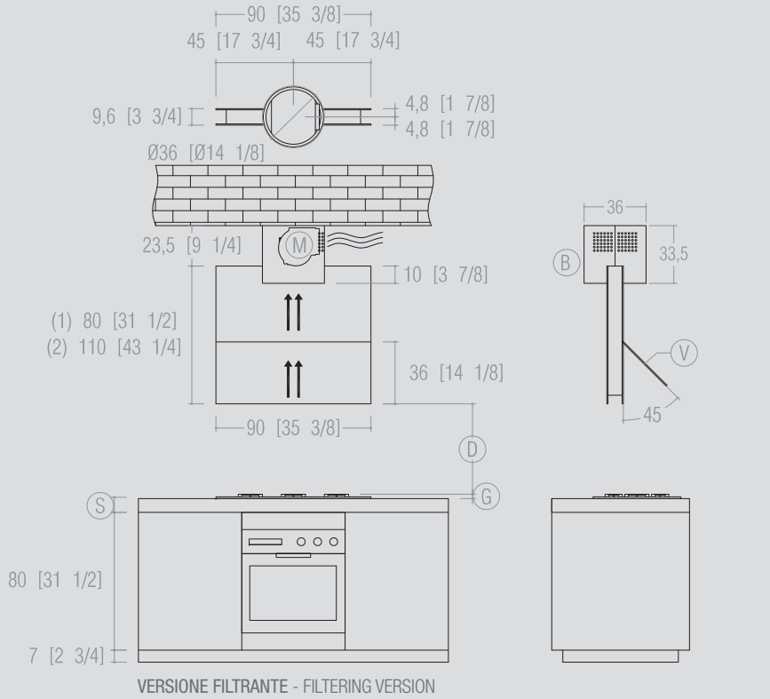
VERSIONE FILTRANTE - FILTERING VERSION
