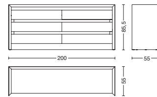
Cod. SOFTWOOD 2 L. 200 - P. 55 - H. 85,5
