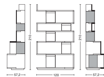
Cod. VAMIZI SMALL L. 120 - P. 57,2 - H. 210
