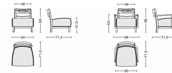
Cod. WILMA L. 64 - P. 41,5 - H. 68
