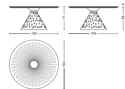
Cod. COLINO R1 Ø. 150 - H. 71
