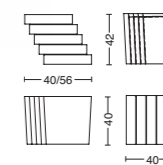
J+I SHIFT Design: Tomoko Azumi Cod. J+I SHIFT L. 40/56 - P. 40 - H. 42
