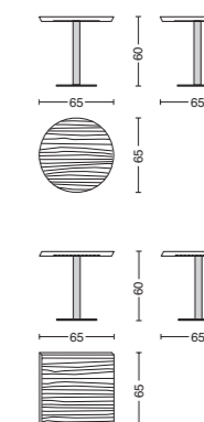
Cod. PEBBLES TONDO Ø 65 - H. 60
