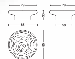
Cod. KENOBI_SMALL TABLE Ø. 79/85 - H. 30
