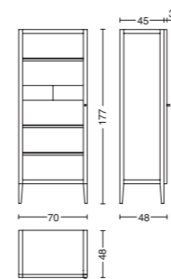
Cod. LIGHT SMALL L. 70 - P. 48 - H. 177
