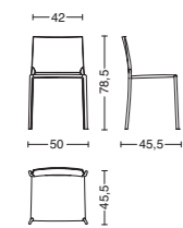
Cod. KAU L. 50 - P. 45,5 - H. 78,5
