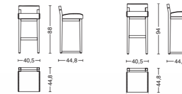
DINO 1 L. 40,5 - P. 44,8 - H. 88
