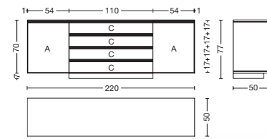
Cod. KYOTO 2013.1 L. 220 - P. 50 - H. 77
