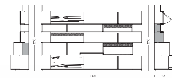
Cod. VAMIZI TV WALL L. 320 - P. 57,2 - H. 210
