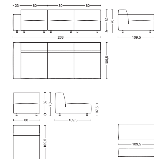
Cod. SKIPPER 3.1BL L. 263 - P. 109,5 - H. 37,5/70
