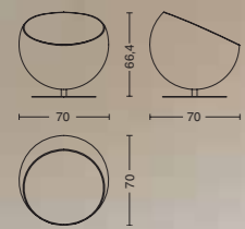
Cod. GLOBE CHAIR L. 70 - P. 70 - H. 66,4
