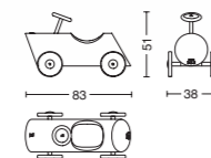
Cod. R313 MICRO L. 83,2 - P. 38 - H. 50,8
