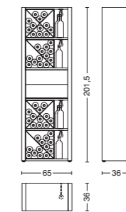
Cod. CRU COMPOS. 2 L. 65 - P. 36 - H. 201,5
