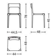
Cod. SLEEK CHAIR L. 44,5 - P. 48 - H. 78
