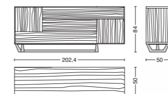
Cod. DAFNE L. 202,4 - P. 50 - H. 84
