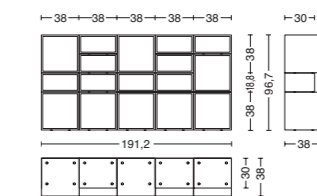
Cod. FREEDOM PROJECT 2 L. 191,2 - P. 30/38 - H. 96,7
