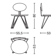
Cod. DAGDA L. 55,5 - P. 53 - H. 80
