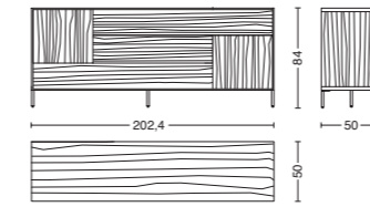
Cod. DAFNE 1 L. 202,4 - P. 50 - H. 84
