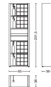
Cod. CRU COMPOS. 1 L. 65 - P. 36 - H. 201,5
