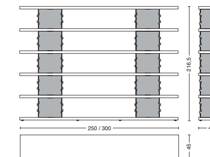
Cod. BRIE-COMP2 L. 250/300 - P. 45 - H. 216,5
