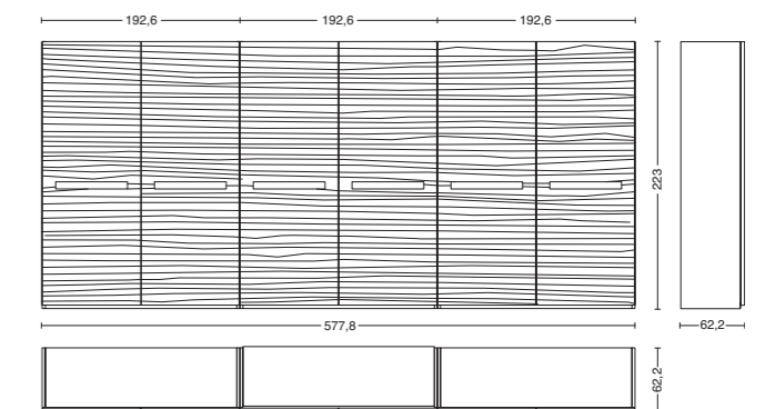
Cod. PLANO 3 L. 577,8 - P. 62,2 - H. 223
