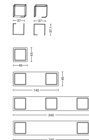
Cod. TUBULAR_FRAME 1 L. 37 - P. 37 - H. 37
