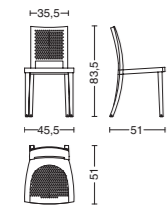
Cod. ARB PIMPINELL 7 L. 45,5 - P. 51 - H. 83,5
