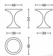
Cod. MURITAZE Ø. 49 - H. 54
